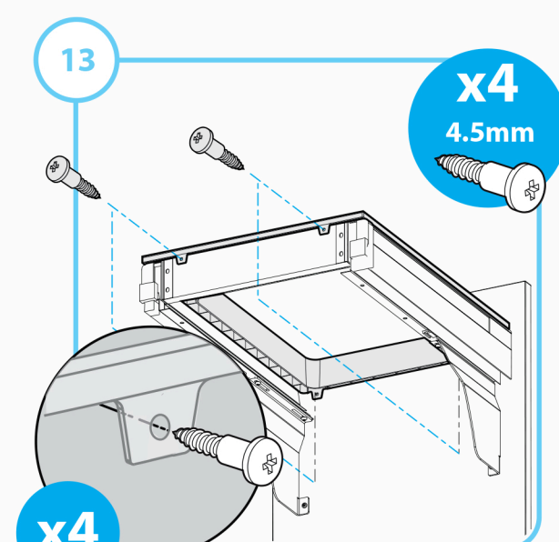
Fixer le plateau avec les vis d'axe
