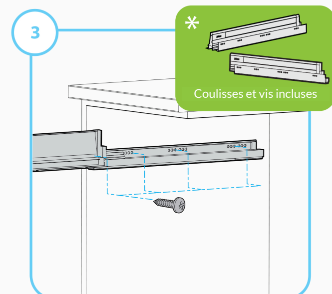
Installer les coulisses selon les spécifications du fabricant
