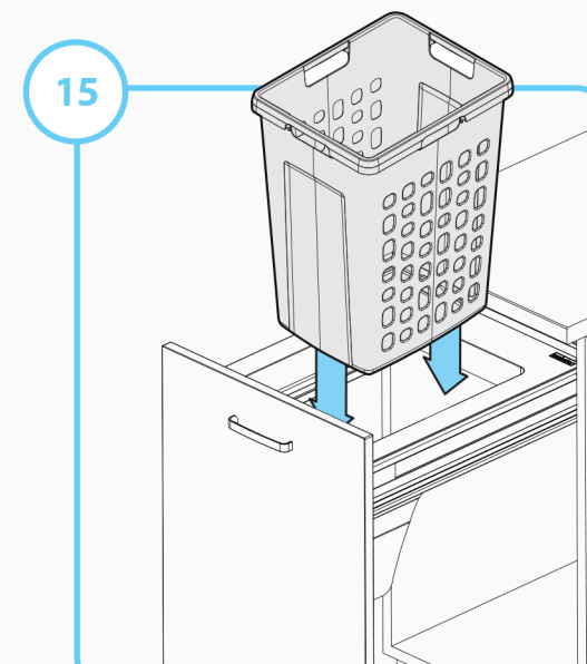
Mettre le panier en place
