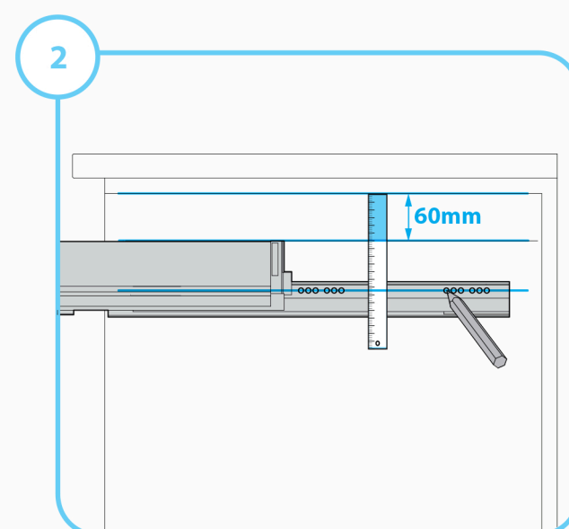
Mesurer 60 mm (minimum) au-dessus du côté et marquer les trous de la coulisse
