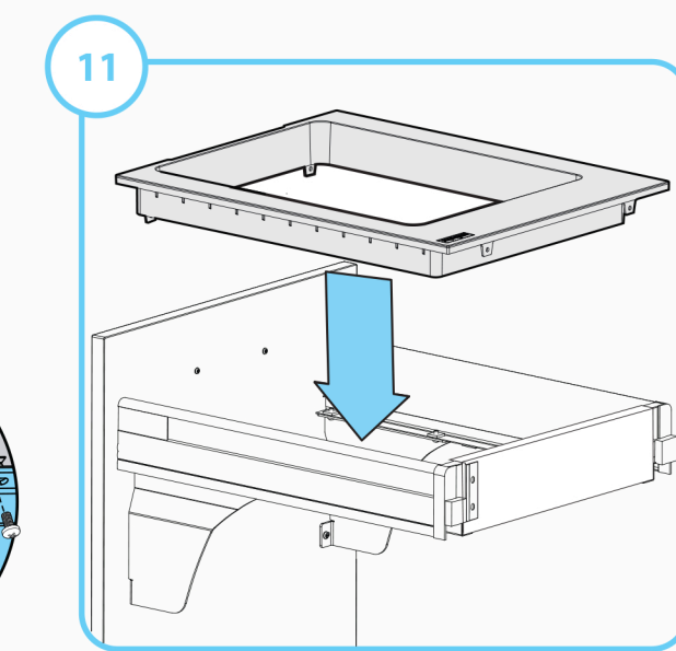
Installer le plateau
