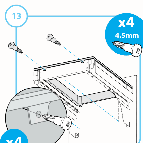
Fixer le plateau avec les vis d'axe
