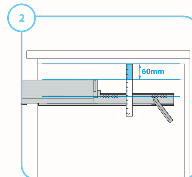
Mesurer 60 mm (minimum) au-dessus du côté et marquer les trous de la coulisse
