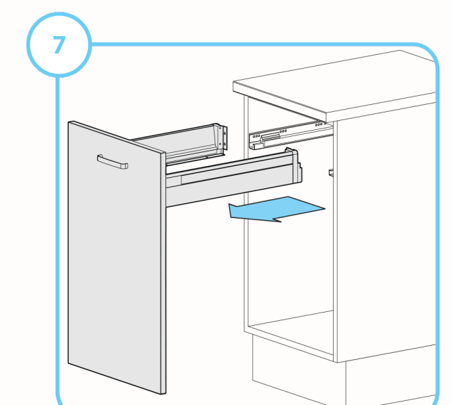
Enlever le tiroir
