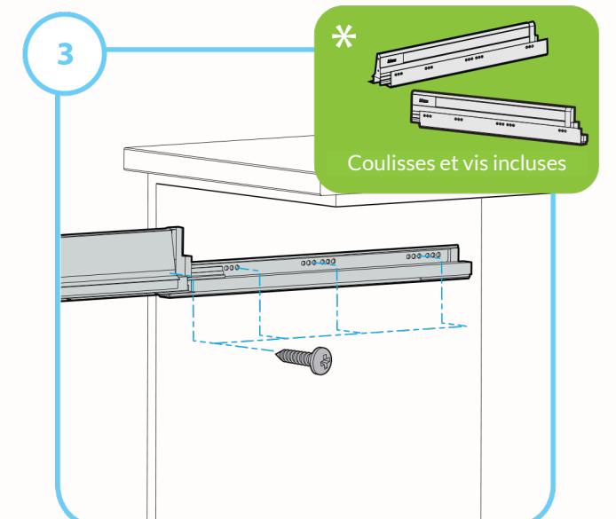
Installer les coulisses selon les spécifications du fabricant
