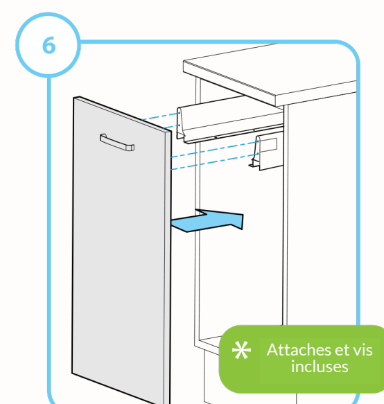
Fixer les attaches de façade sur la porte et clipser sur les côtés
