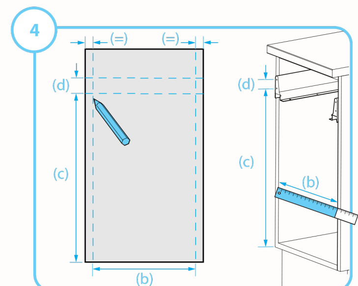
Mesurer la largeur du caisson (b), la hauteur des trous de la coulisse (c), et l'espacement (d) et transposer sur la porte
