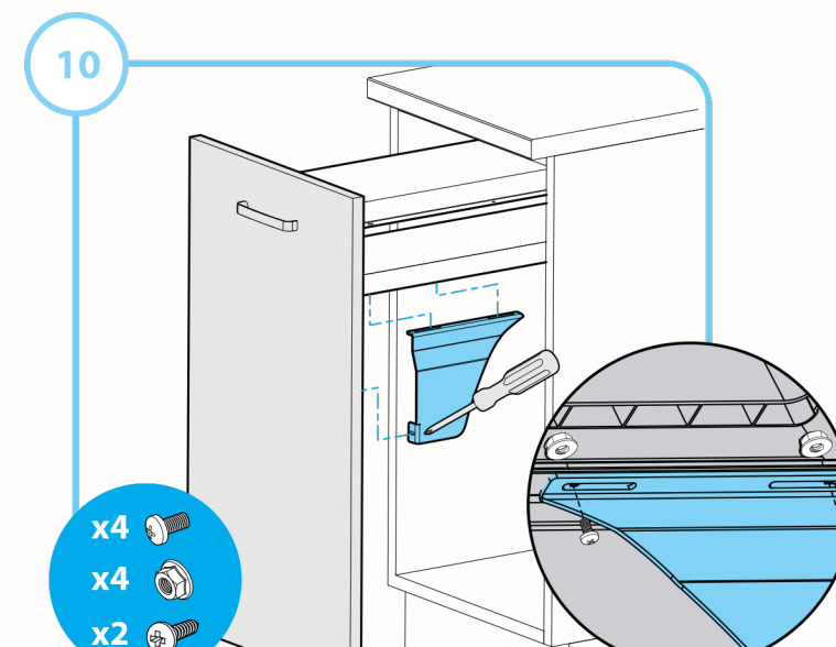
Fixer les équerres de maintien de la porte
