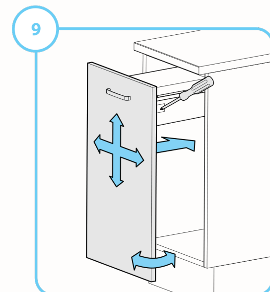
Réinstaller le tiroir et ajuster la porte
