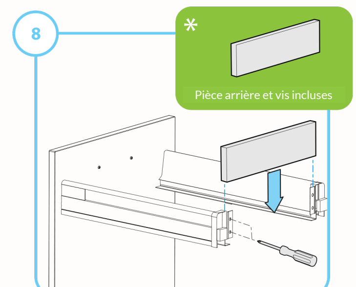
Installer le dos du tiroir selon les indications du fabricant
