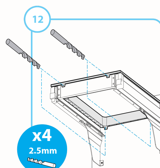
Centrer le plateau, marquer et percer les trous
