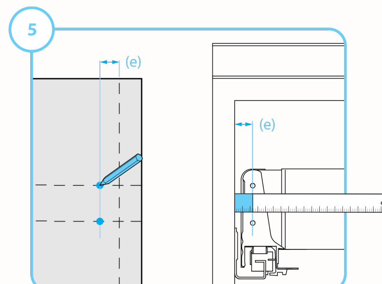
Mesurer la distance des attaches de façade et marquer la porte
