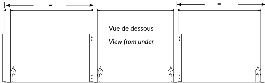
Coulisse Dynapro BM 40 kg réparties à distance égales sous le tiroir. 40 kg Dynapro BM placed equally on the drawer bottom.
