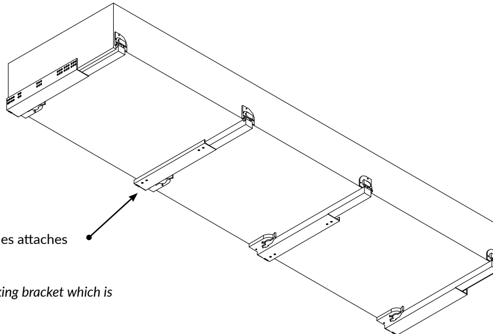
Coulisse Dynapro BM 40 kg réparties à distance égales sous le tiroir. 40 kg Dynapro BM placed equally on the drawer bottom.
